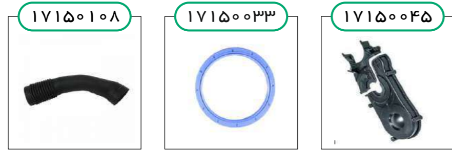
۱۷۱۵۰۱۰۸ کانال خرطومی هواکش پراید ۱۷۱۵۰۰۳۳ کاسه نمد عقب میل لنگ پراید ۱۷۱۵۰۰۴۵ قاب تسمه تایم کوچک پراید مجاری تهویه پراید کبریا ختم العمود المرفقی الخلفی فخر باطار توقيت صغير Pride ventilation duct Pride rear crankshaft seal Pride small timing belt frame
