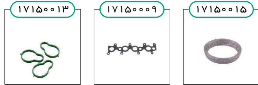
۱۷۱۵۰۰۱۳ واشر منیفولد هوای پراید یورو ۴ مجاری تهویه پراید Euro 4 Pride Air Manifold Washer ۱۷۱۵۰۰۰۹ واشر منیفولد هوای پراید غسالة براید مشعب الهواء Pride Air Manifold Washer ۱۷۱۵۰۰۱۵ واشر گلوبی گرد پراید گرافیتی غسالة حلق دائرية من براید جرافیتی Exhaust seal gasket (rounded graphite)
