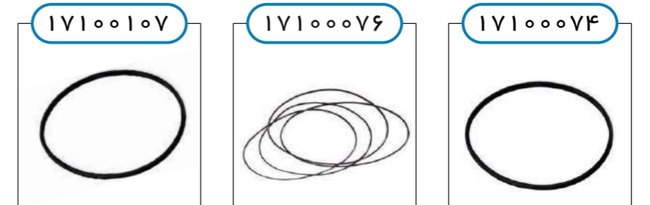
اورینگ دوراهی آب پشت سرسیلندر ۴۰۵ تقاطع المياه الدائری، الجزء الخلفی من رأسی الأسطوانة water intersection O-ring, rear of the cylinder head اورینگ دور بوش پژو ۴۰۵ بوش یا الدائری Cylinder liner O-RING اورینگ درجه داخل باک ۴۰۵ هفت درجه الوقود یا الدائری الصف FUEL GAUGE O-RING
